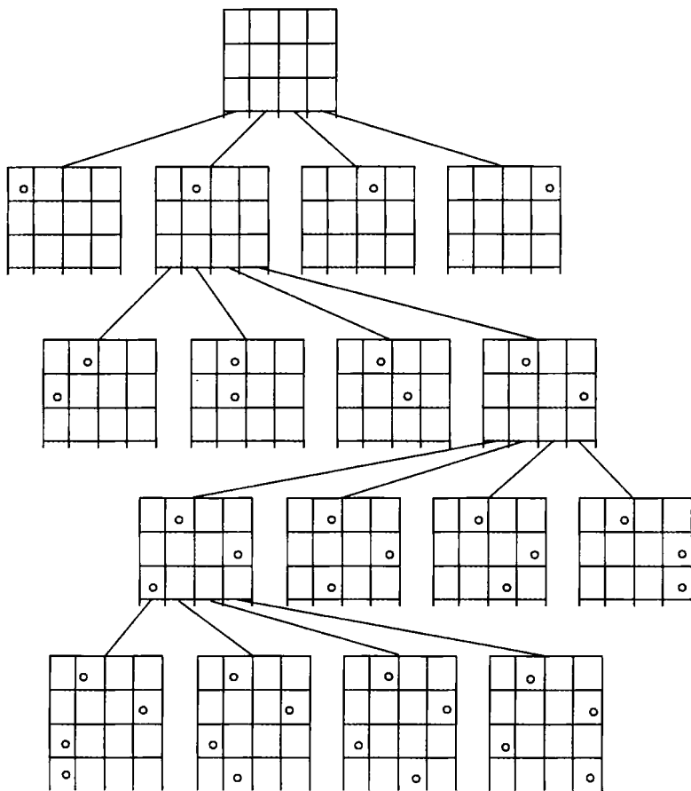
图 1.2 四皇后问题中隐含的状态树
