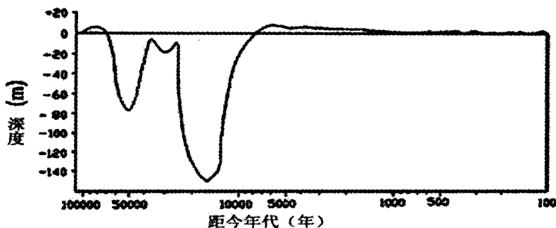
海平面升降曲线图②
