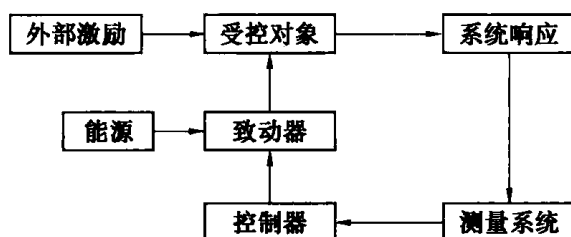
图 1.2 反馈主动控制系统
