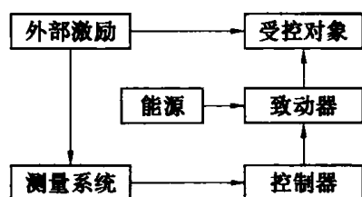
图 1.1 前馈主动控制系统
