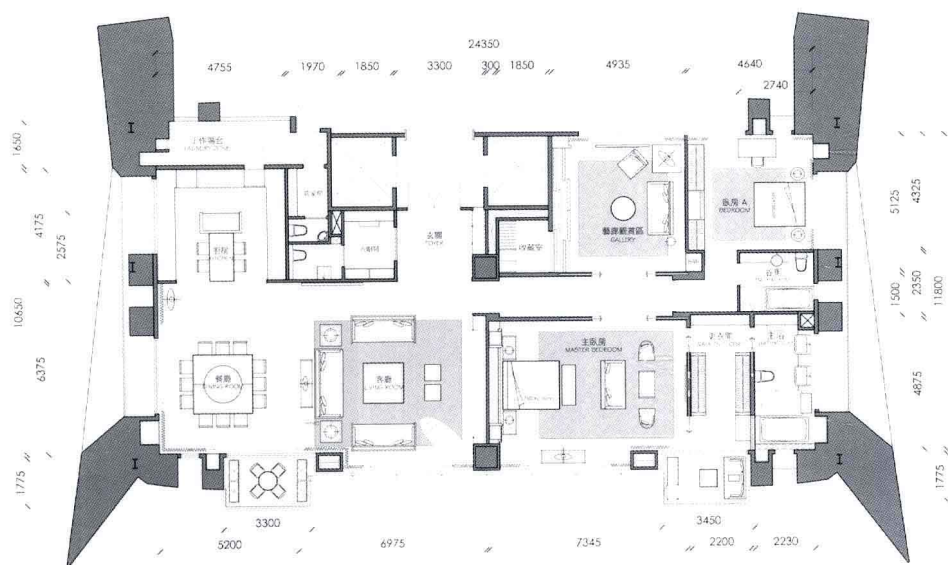
平面布置图
