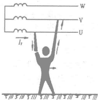
图 1-3 两相触电
