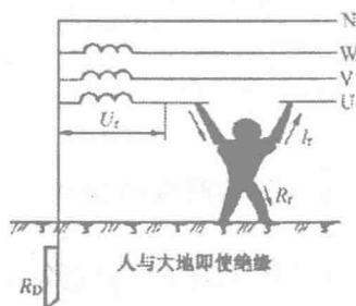
图 1-2 单相触电的另一种形式
