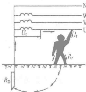
图 1-1 单相触电的一种形式
