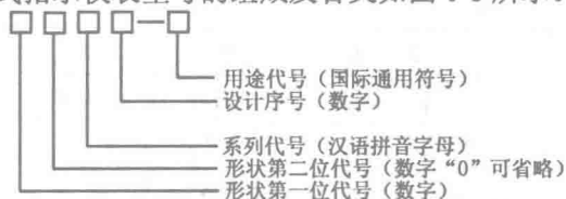
图 1-8 安装式指示仪表型号的组成
