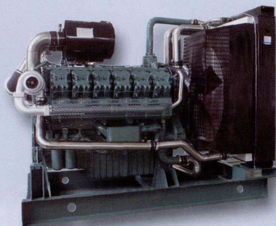
新推出追赶国际先进水平的 “蓝迪”系列大功率柴油机
