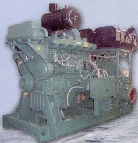
万迪138系列柴油机泵类配套机组
