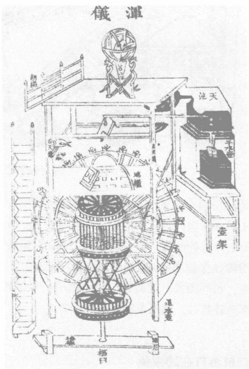
水运仪象台图
