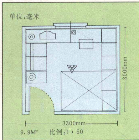
▼多功能小卧室室内设计平面图
