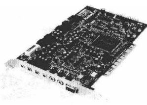
图 1.7.7 声卡
