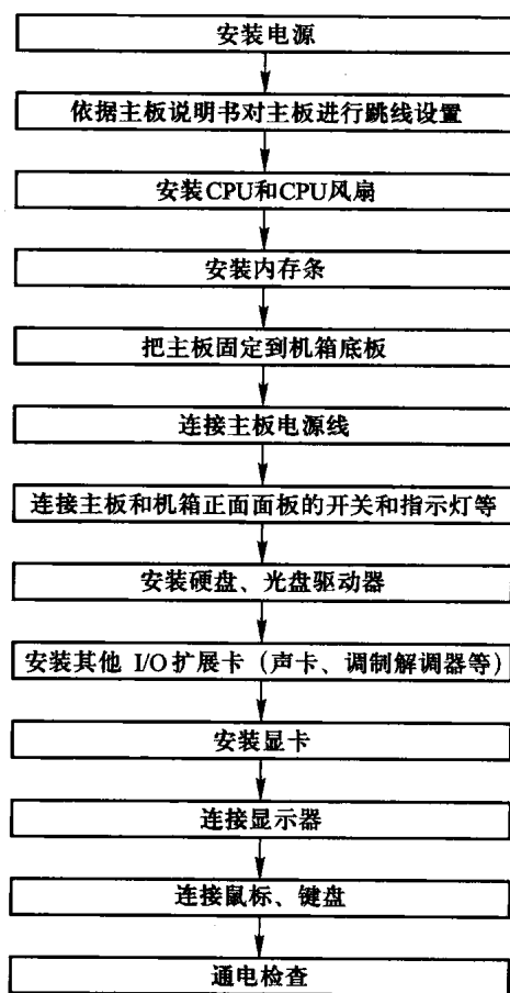
图 1.4.1 微型计算机组装流程图
