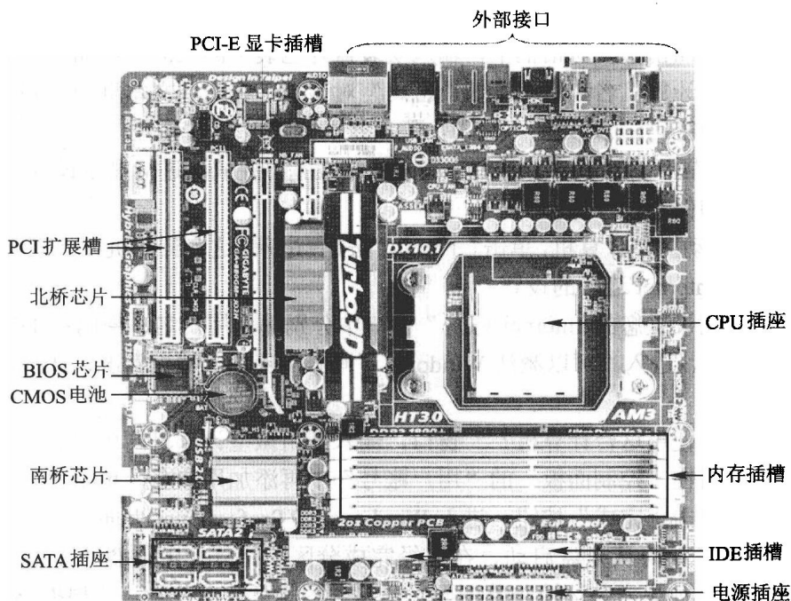
图 1.7.4 主板
