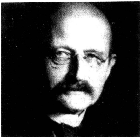
德国著名物理学家马克斯·普朗克。1900年提出“量子假说”，对量子论的发展有重大影响。
