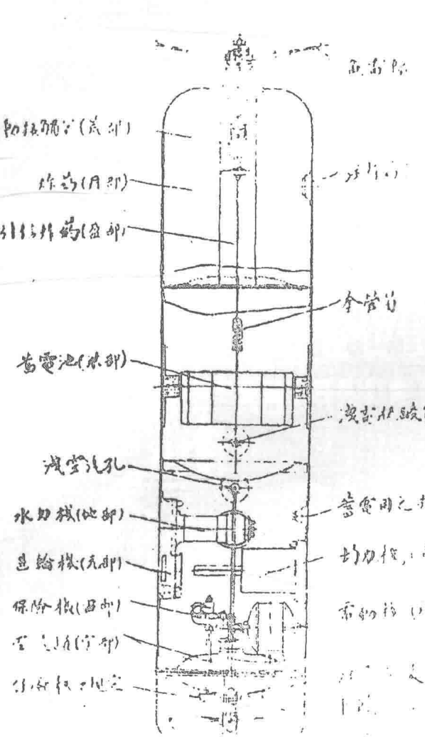
德國電氣魚雷切面圖形
