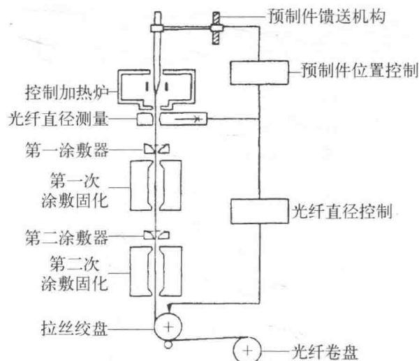
图 1.5 光纤拉丝工艺
