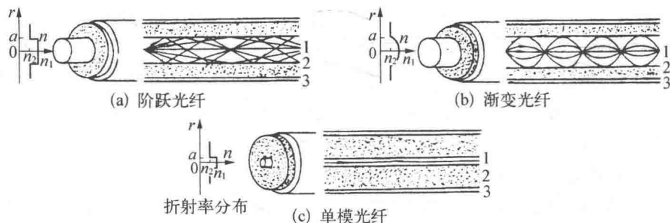
图 1.1 光纤的结构
