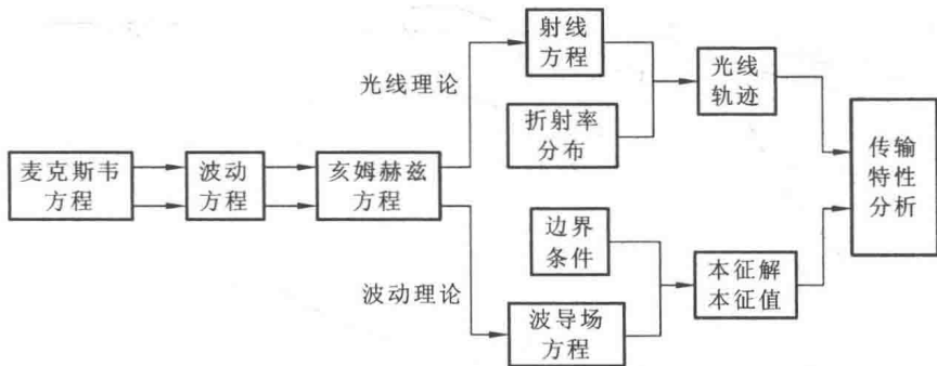
图 2.1 光线理论与波动理论分析思路
