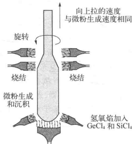
图 1.4 VAD 预制棒工艺
