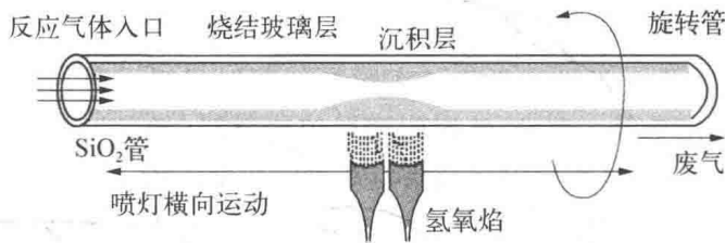
图 1.2 MCVD 预制棒工艺
