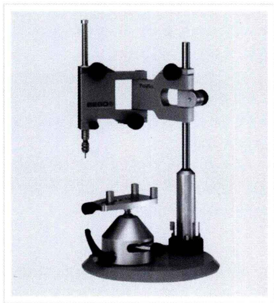
图 1-6 模型观测器用来确认牙列中有关基牙的长轴与义齿就位道之间的关系，是设计制作可摘局部义齿不可缺少的重要工具
