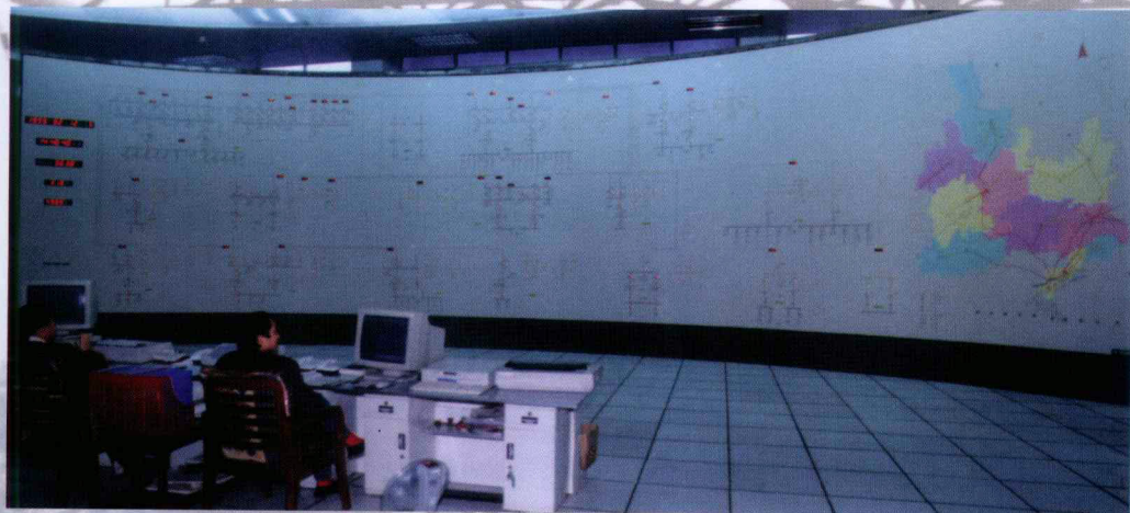
铜仁供电局调度中心
