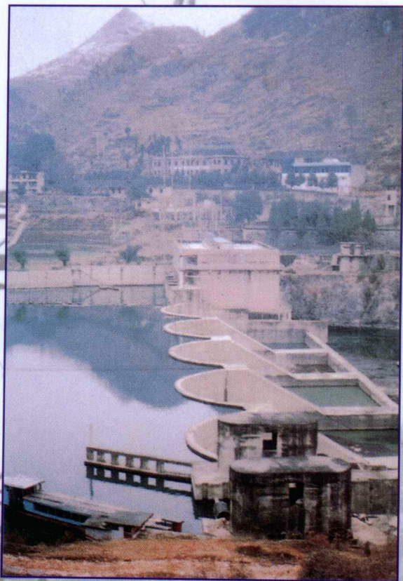
铜仁芦家洞电站（近为船闸）
