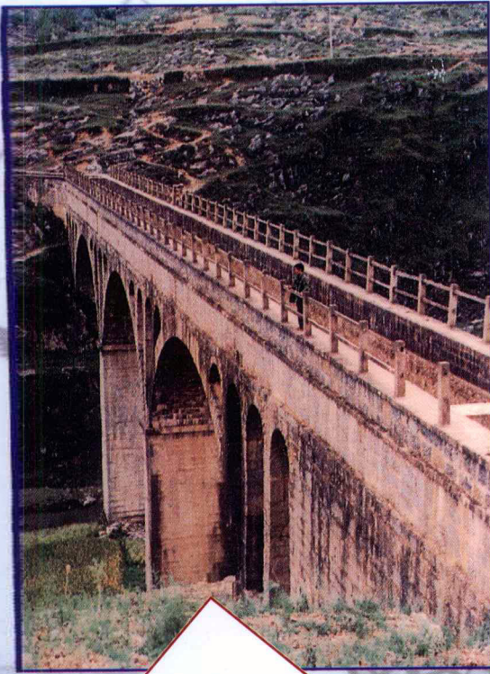
沿河官舟水库跳墩石拱渡槽
