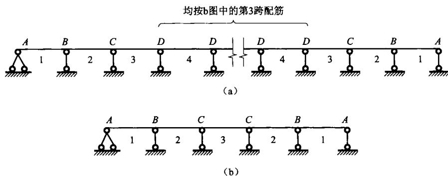
图 8.10 连续梁(板)计算简图
