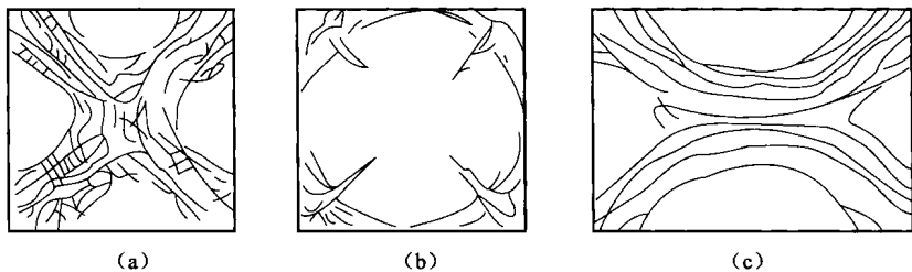
图 8.4 双向板的裂缝示意图
