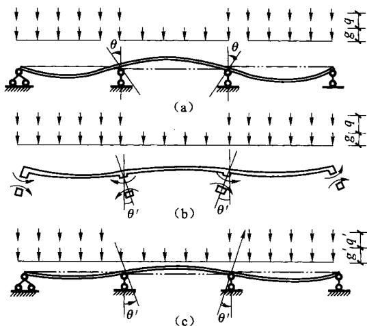
图 8.12 连续梁(板)的折算荷载
