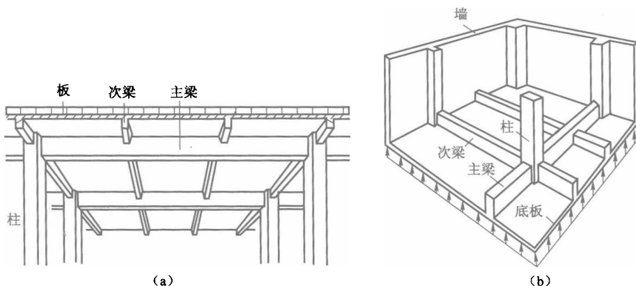
图 8.5 梁板结构
