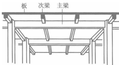
图8.1 肋形楼盖
