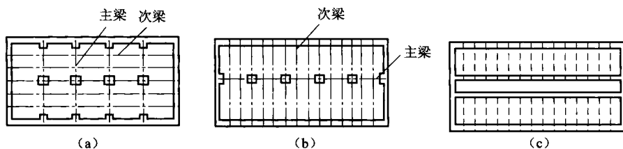
图 8.9 单向板肋梁楼盖结构布置
