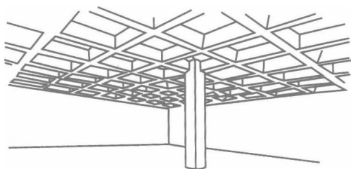
图 8.6 井式楼盖
