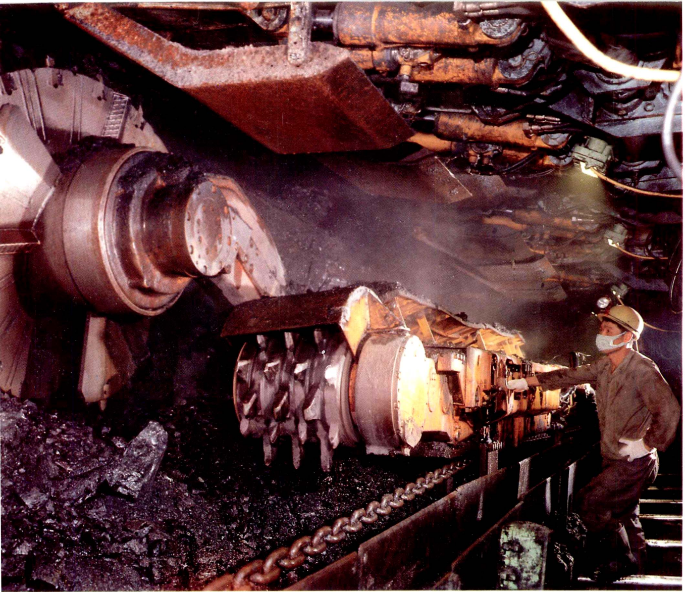
安州地区煤矿联合企业采煤场
