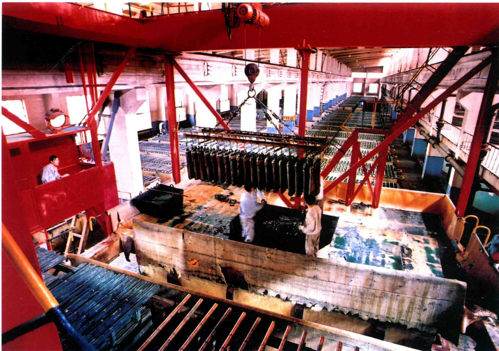
中国镍都金川：金川有色金属公司规模宏大的镍电解厂
