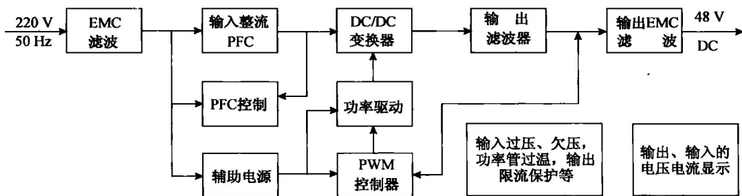
图 1.1.1 开关电源方框图
