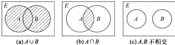
图 1.1 集合 A, B 的并集、交集、两集合不相交
