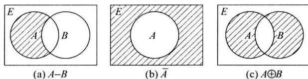
图 1.2 A-B, \bar{A}, A \oplus B 的文氏图
