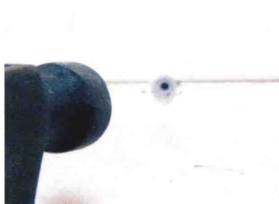
05 壁虎完全钉入洞中的情形。若洞不够深，挂的作品又不会太重时，可以用美工刀把露出来多余的壁虎割除。
