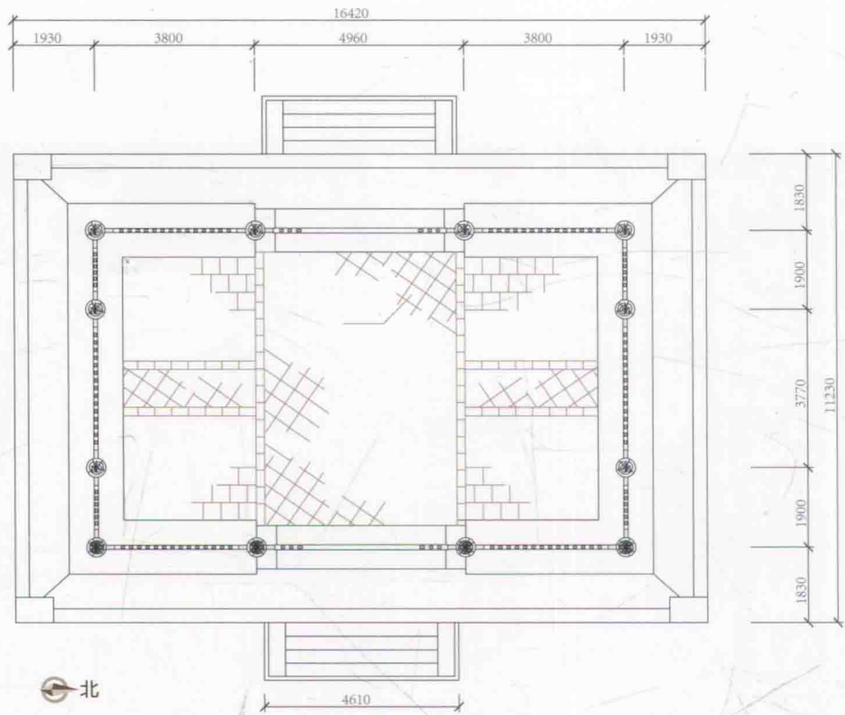
晋祠献殿平面图
