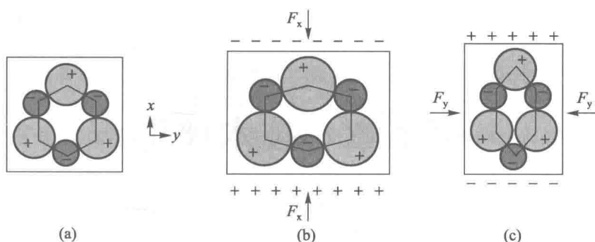
图 1-1 石英晶体的压电传感示意图
