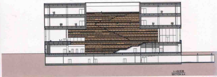
剖面图
