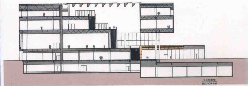
剖面图
