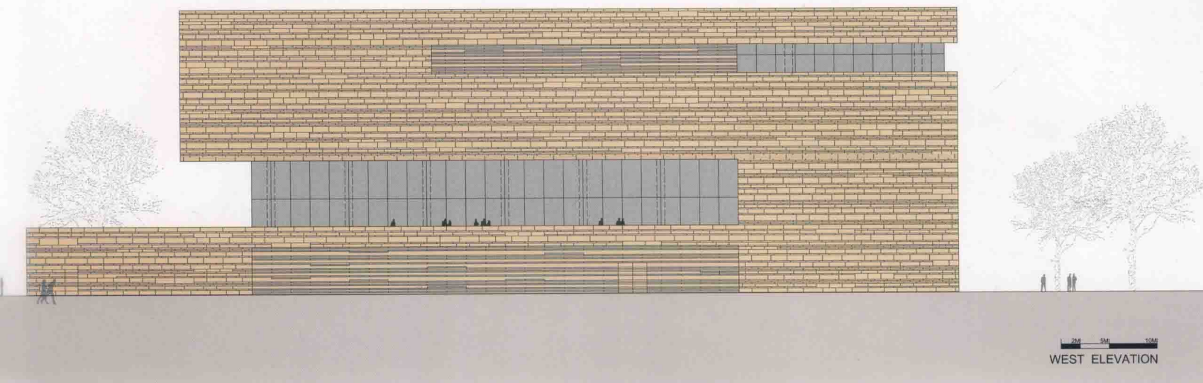
西立面图
