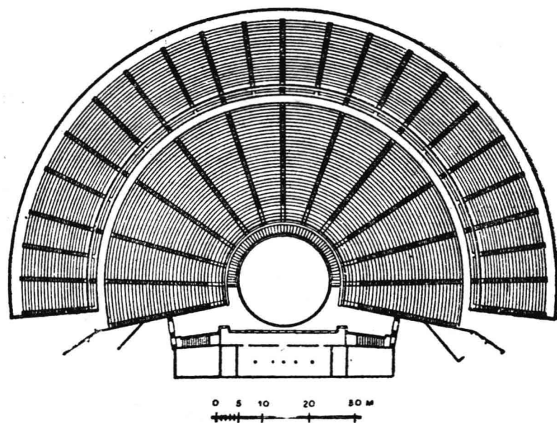
圖6 古希臘埃庇達魯斯劇場平面
