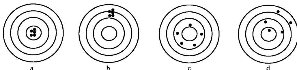
图 1.1 用打靶作比喻展示准确性与精确性的关系
