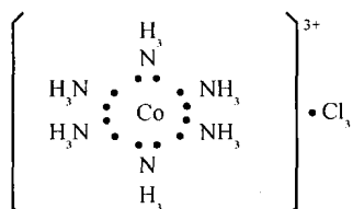
图 1.1 [\text{Co}(\text{NH}_3)_6]\text{Cl}_3 的 Lewis 结构
