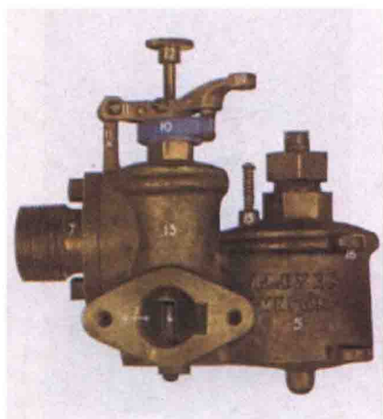
图 1-15 早期化油器
