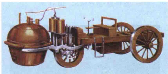
图1-4 居纽研制的蒸汽驱动的汽车
