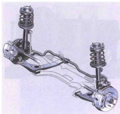
图 1-19 扭力杆式减振器
