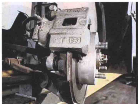
图 1-18 盘式制动器
