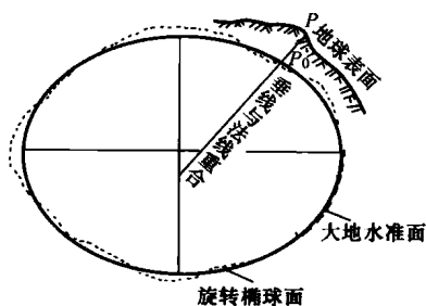
图 1-2 大地水准面和旋转椭球体
