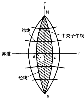
图 1-5 高斯投影展开图
