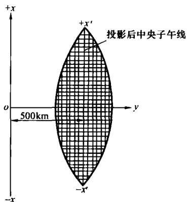
图 1-7 坐标纵轴西移
