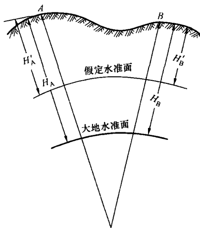
图 1-10 高程示意图
