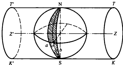
图 1-4 横圆柱投影
