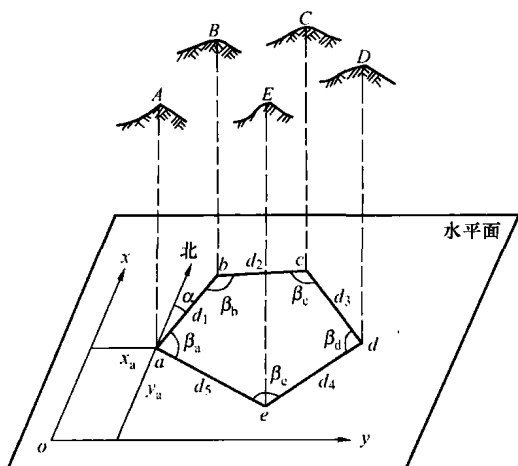
图 1-8 水平面投影
