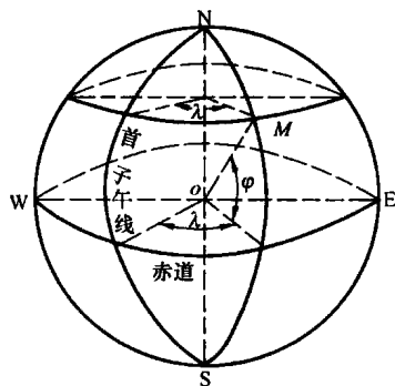
图 1-3 地理坐标
