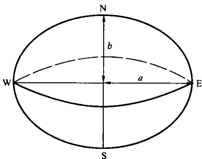
图 1-1 旋转椭球体
