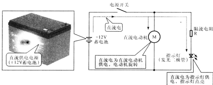
图 1-1 典型的直流供电电路
