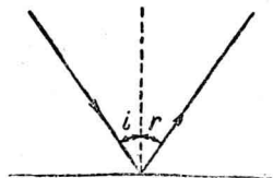
圖 3. 反射定律底示意圖。
