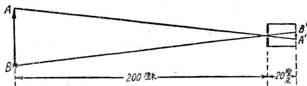
圖 2. 光底直線傳播: 用一個小孔成像。
