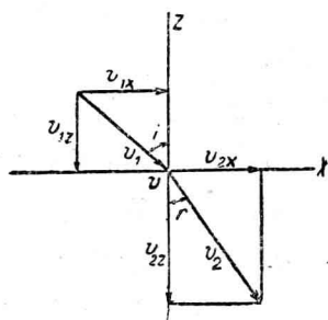
圖 4. 折射定律底示意圖。
