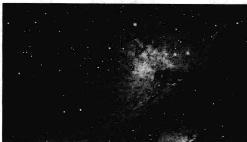
美丽的猎户座大星云
