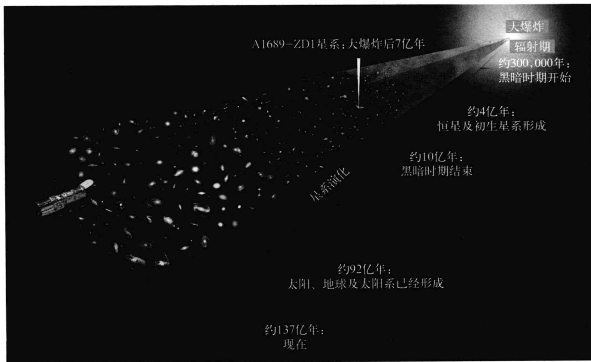
宇宙大爆炸演化示意图(即宇宙纪元示意图)
