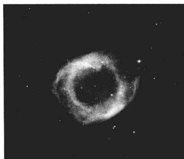
宝瓶座“上帝之眼”螺旋星云
