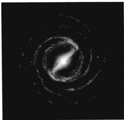
银河系的正面图
