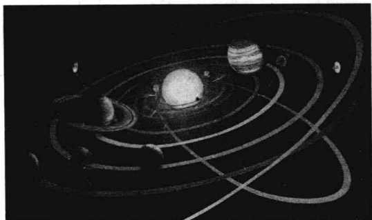
太阳系的运行图
