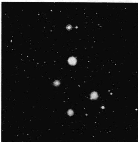
宿星团是 7800 万年前从气体和尘埃构成的星云中诞生的,在星云残余物的包围中大约有 100 颗星体。
