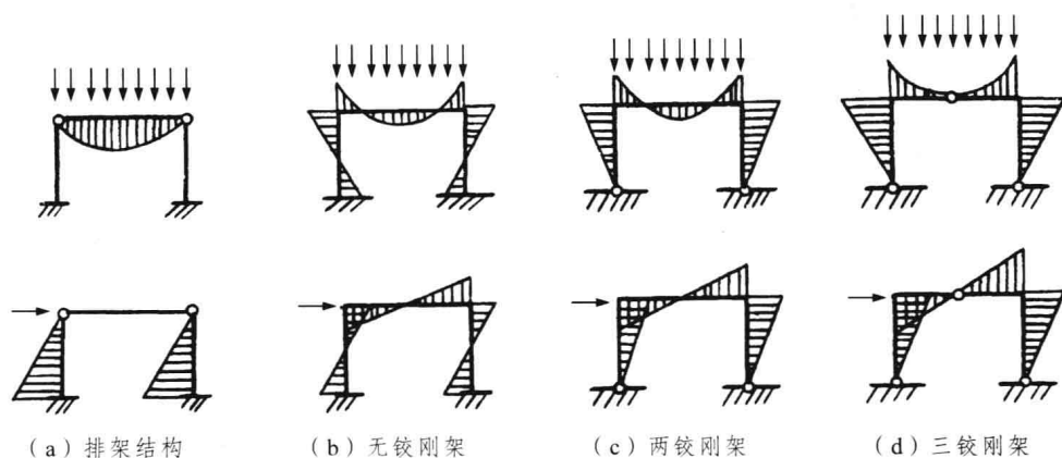
图 1.13 刚性连接与铰接的弯矩比较
