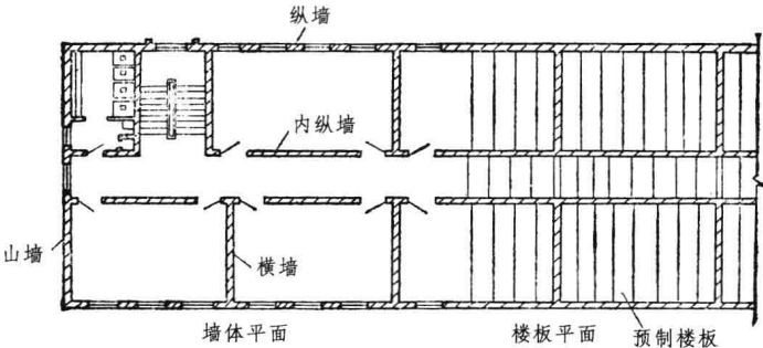
图 1.9 纵墙承重方案
