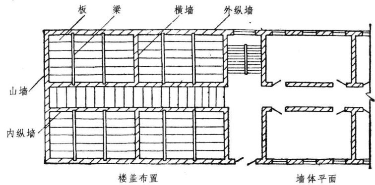
图 1.10 纵横墙承重方案
