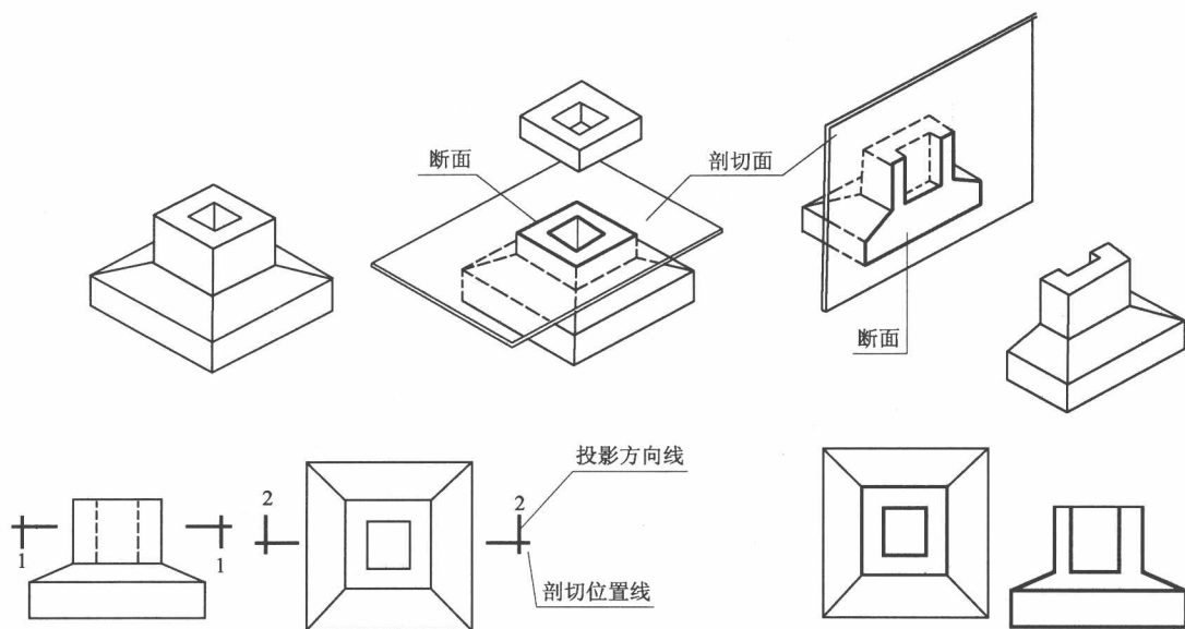
图 1-14 剖面图
