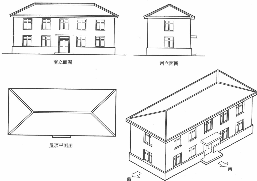
图 1-13 三面正投影图的应用
