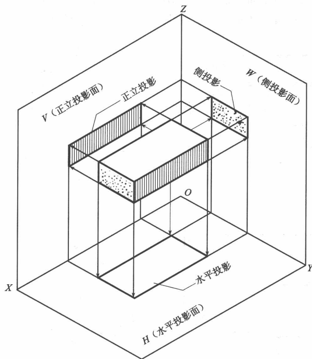
图 1-11 三面正投影图
