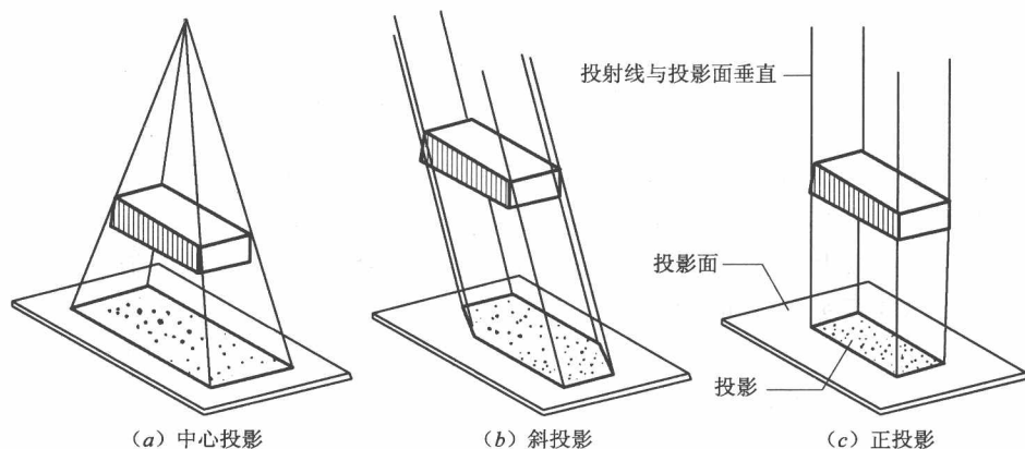
图 1-4 投影的类型
