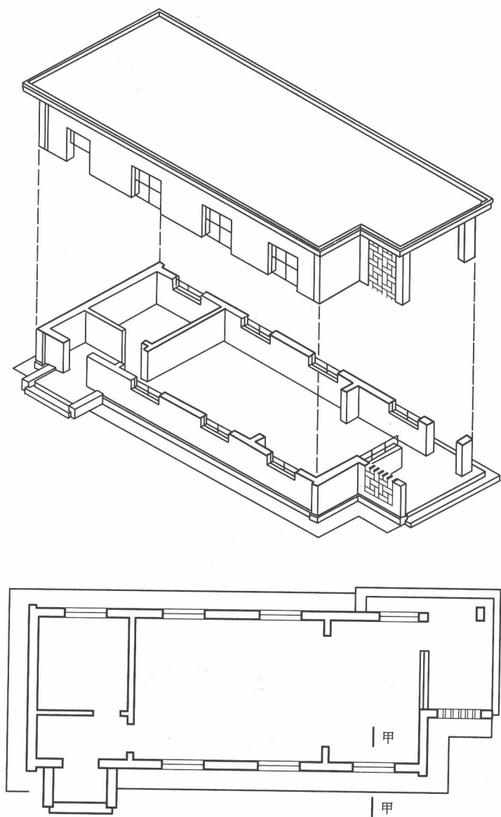
图 1-15 平面图的形成
