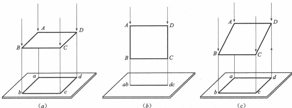
图 1-8 平面的正投影
