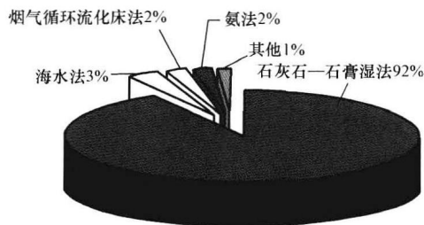
图 1-5 2009 年底前烟气脱硫机组二氧化硫治理方法
