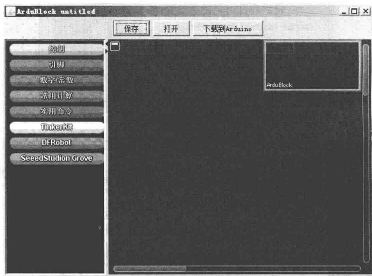
图 1-9 ArduBlock 编辑器
