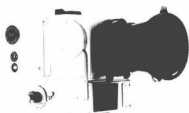
太空电子数据照相机 EDC ——月球照相机
