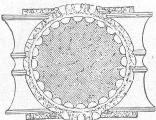
4. 普通依翁里式柱頭之斷面圖
