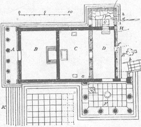
8. 愛里西特翁廟之圖樣
