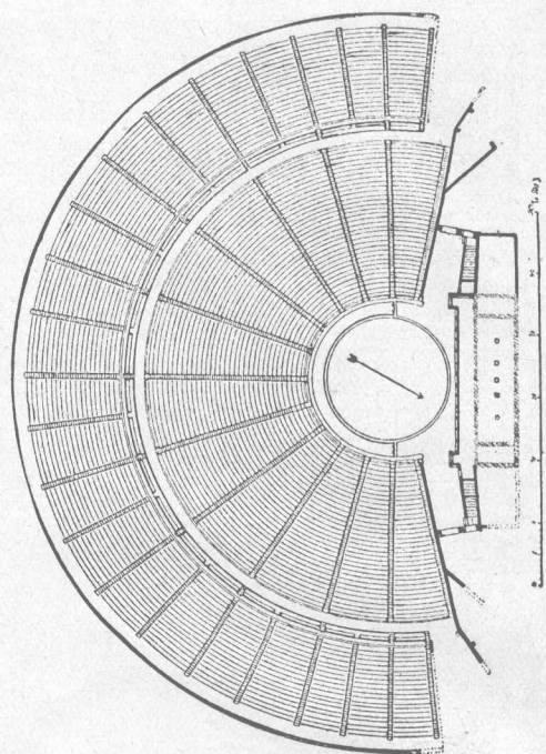
2. 愛皮島羅斯之戲台圖樣
