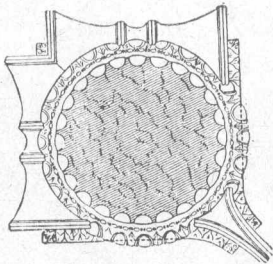
5. 依翁里式角柱頭斷面圖
