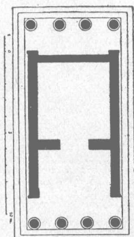
6. 阿非蒲羅斯體諾斯式之地基
