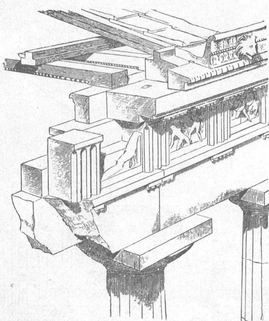
4. 柱頂之承担狀
