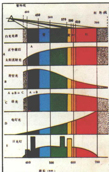
图2 各种光源的光谱。从图中可以看出，电灯光红黄色多，日光灯光谱不全，不宜用彩色片拍摄。
