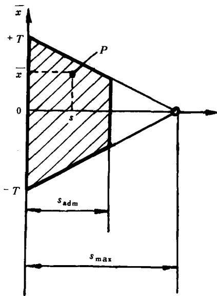
图 3 验收梯形
