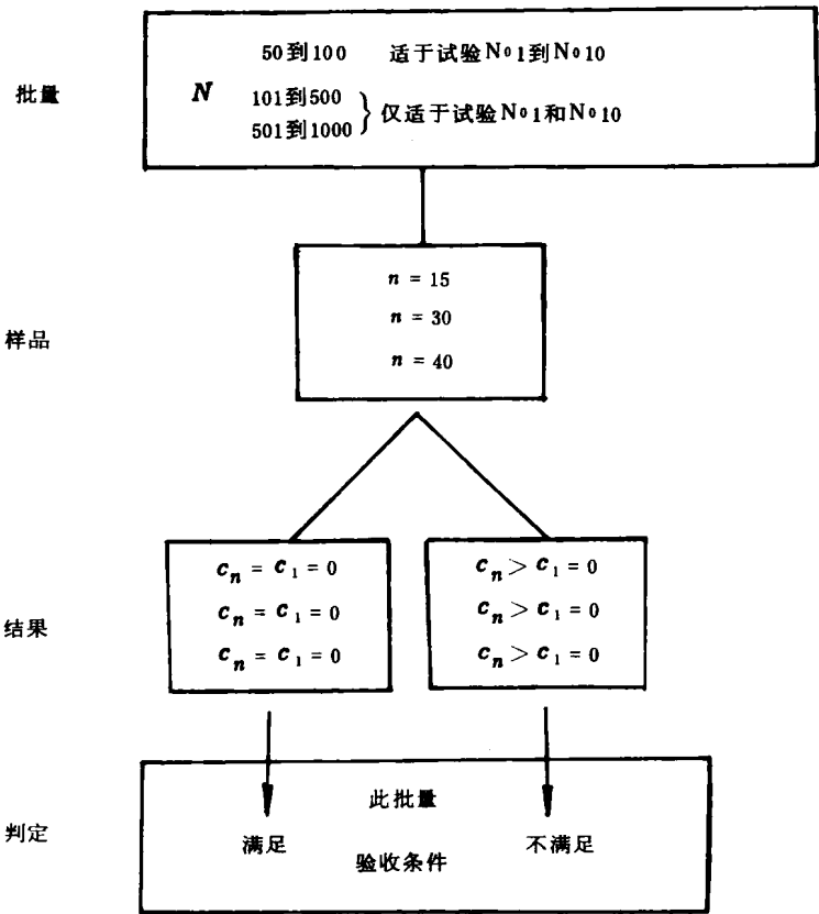
图1 一次抽样图
