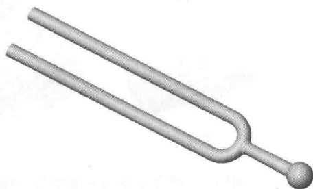
图 1-3 音叉模型
