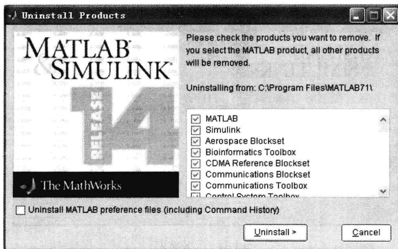
图 1-13 卸载 MATLAB 7
