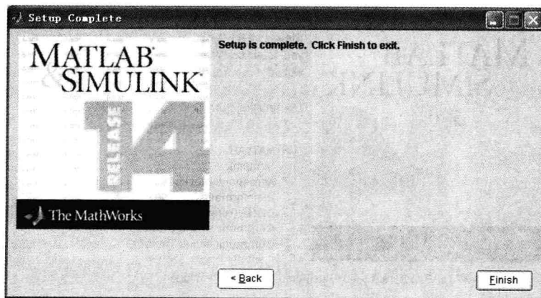
图 1-11 安装结束
