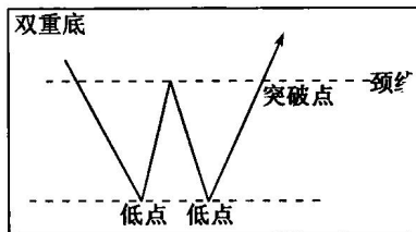
图 1-2 双重底
