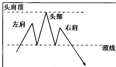
图 1-3 头肩顶
