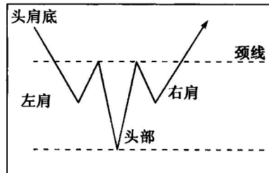
图 1-4 头肩底
