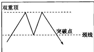
图 1-1 双重顶
