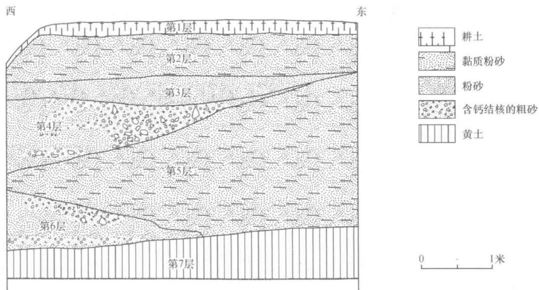
图四 李家沟遗址北区北壁剖面图
