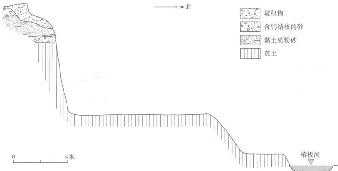
图三 李家沟遗址附近椿板河谷剖面示意图
