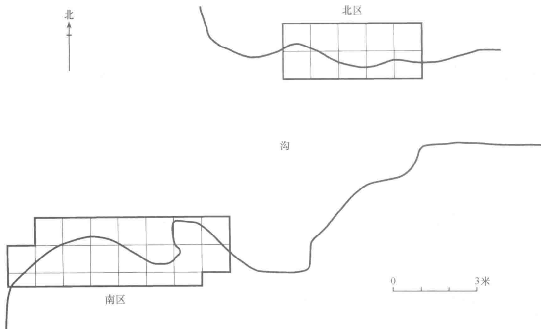
图二 李家沟遗址探方分布图
