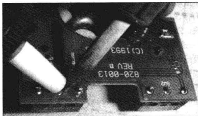
(焊下欧姆龙开关)
