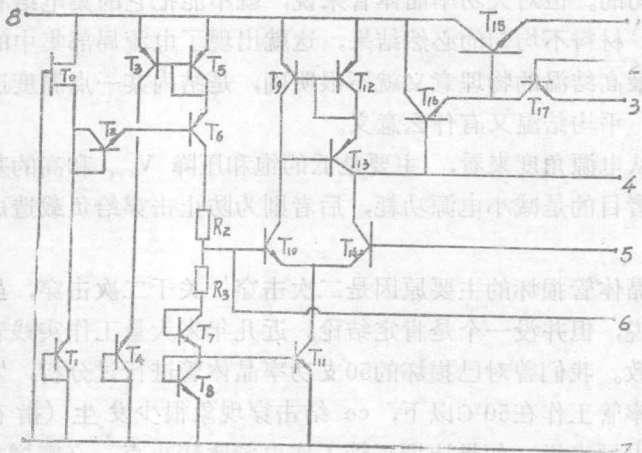
图(二) 5G14电路图
