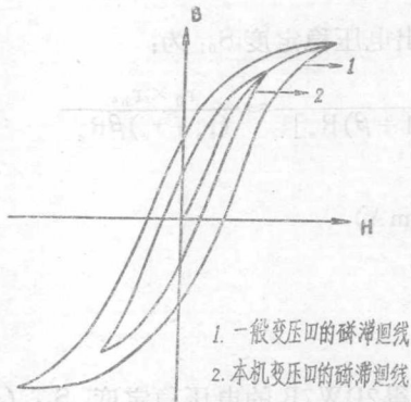
图4. 几种条件下的变压器磁滞回线
