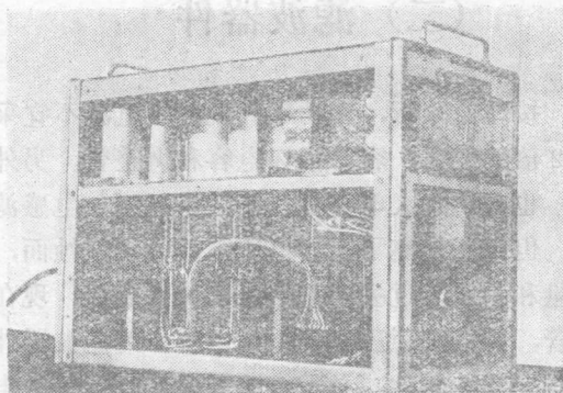
图(一) 电源结构图
