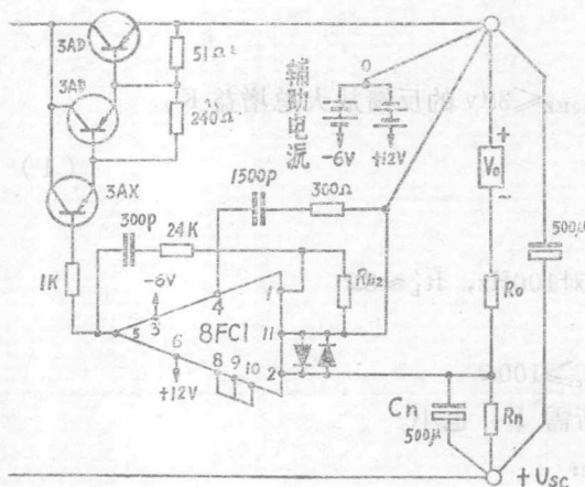
图1 调整管用锗管的电路
