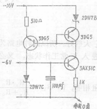
图3 基准电压输出电路
