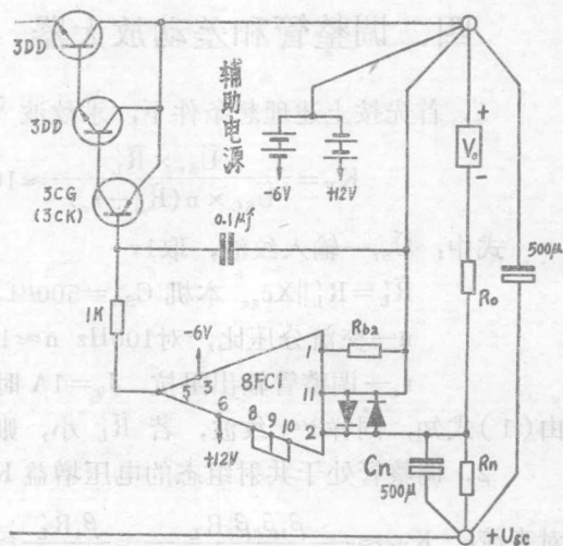
图2 调整管用硅管的电路
