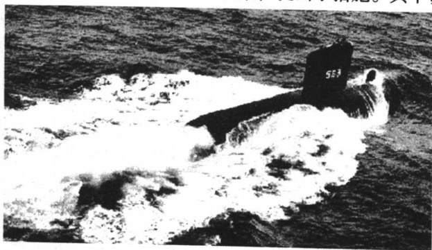
图 1-2 美国第 1 艘水滴型潜艇“大青花鱼”号。它水面排水量 1242 吨，水下排水量 1847 吨，全长 62 米，在美国海军潜艇中属五短身材
