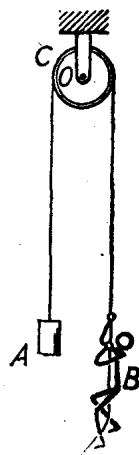
图5.5 适当选取质点系可使外力简化
