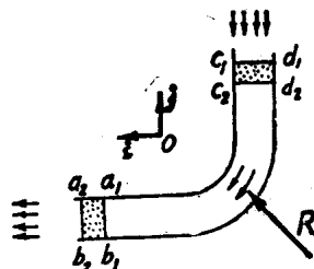
图5.10 弯管反力
