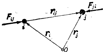
图5.4 内力主矩为零
