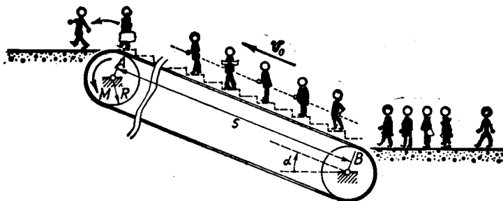
图5.8 求平均力矩 M
