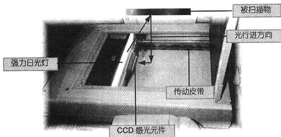
平台式扫描仪工作原理与基本部位
