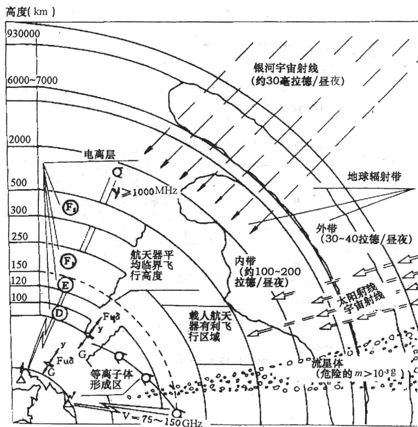
图 1.4 近地宇宙空间的主要因素
