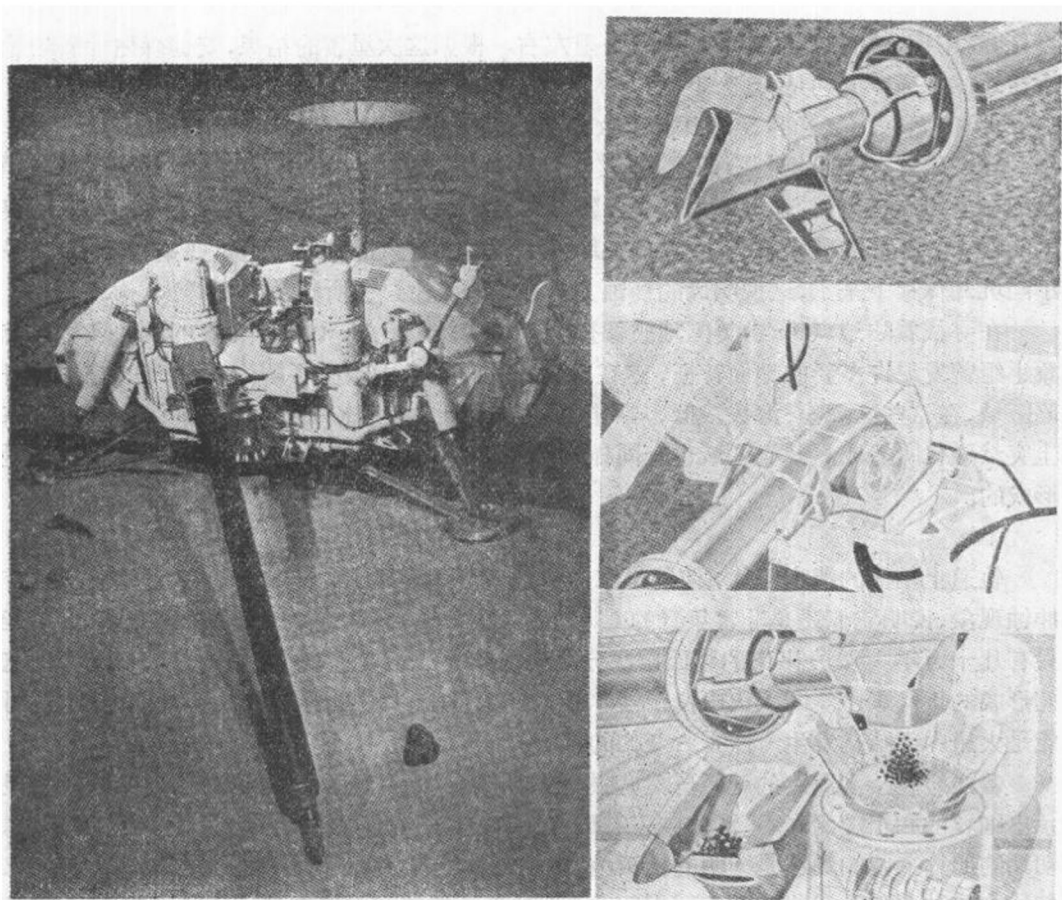
从海盗号着陆舱中伸出一只长的机械手，挖取土样，然后收回，转到一位置，把土样放在小舱内，以进行化学和生物试验
